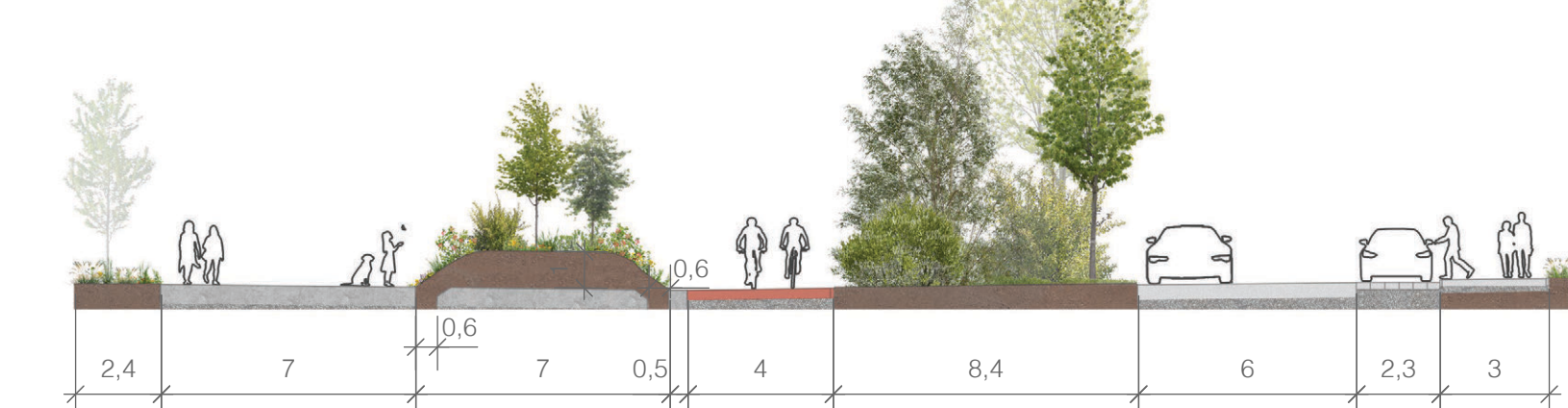
LÕIGE A-A
