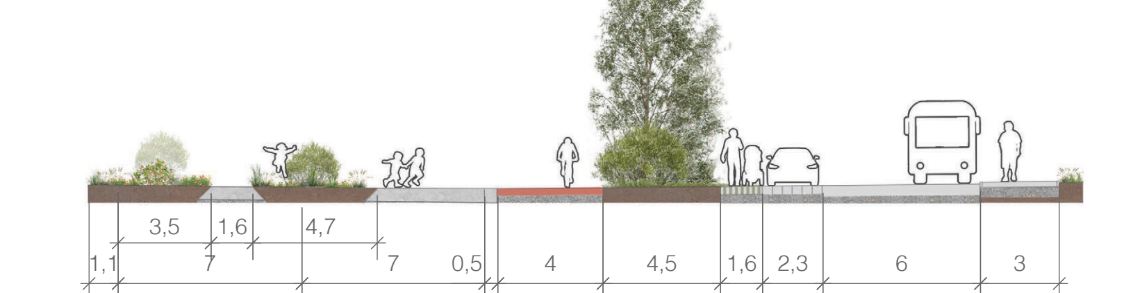
LÕIGE B-B
