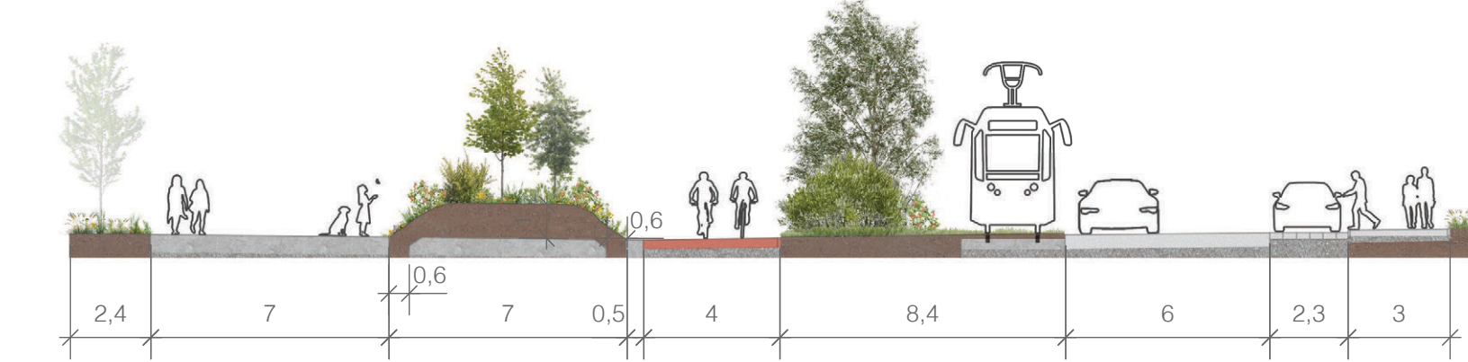
LÕIGE A-A / ALTERNATIIV TRAMMIGA
