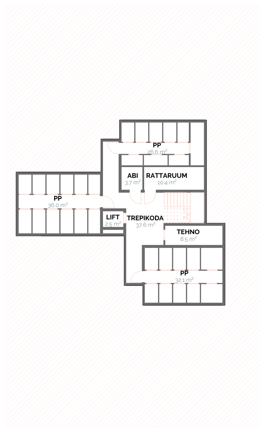
1 T1B KELDRIKORRUS 1 : 200
