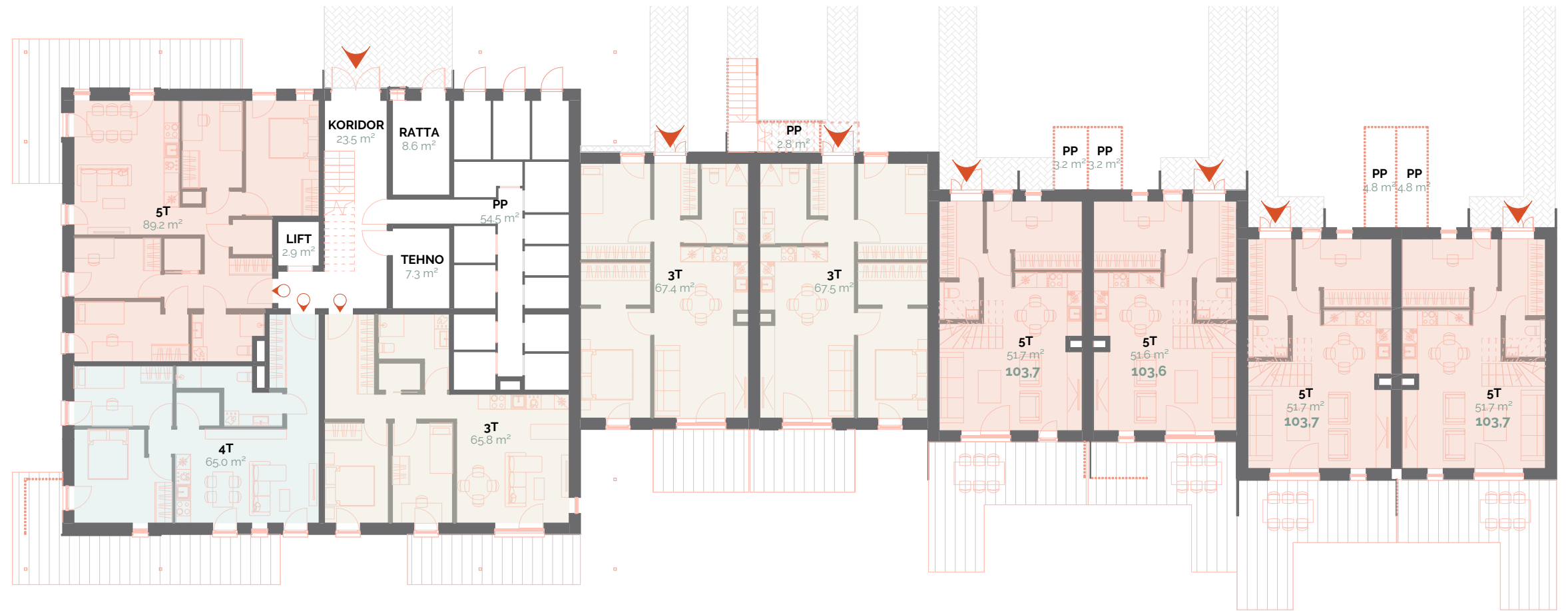
1 T3 + T2B ESIMENE KORRUS 1 : 200
