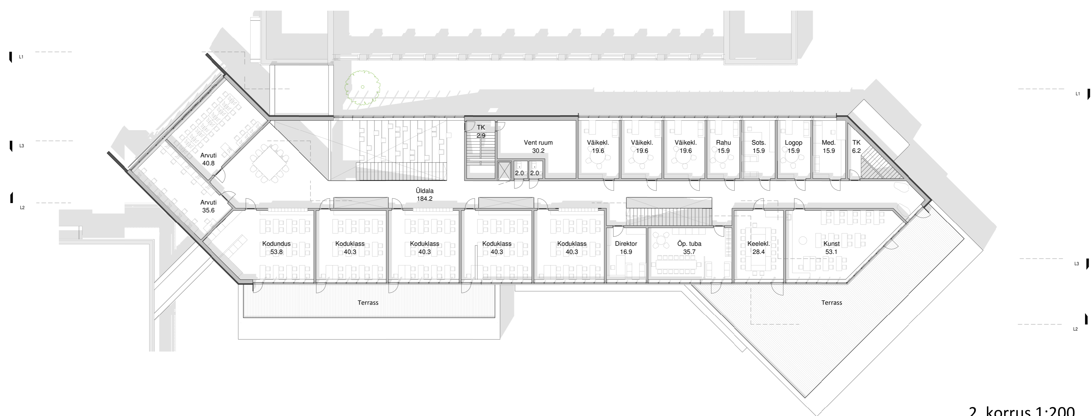
2. korrus 1:200
