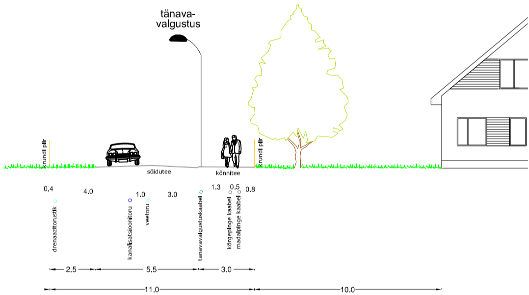
Kavandatud tänava ristprofiil Lõige A-A M 1:200
