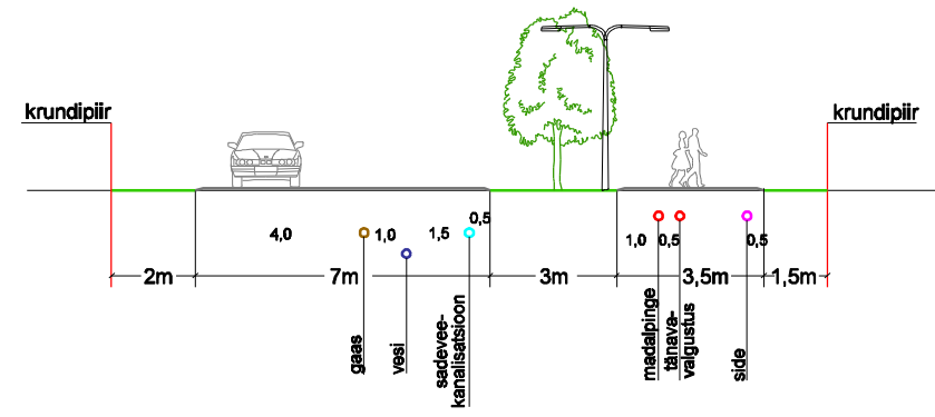
Lõige B - B
