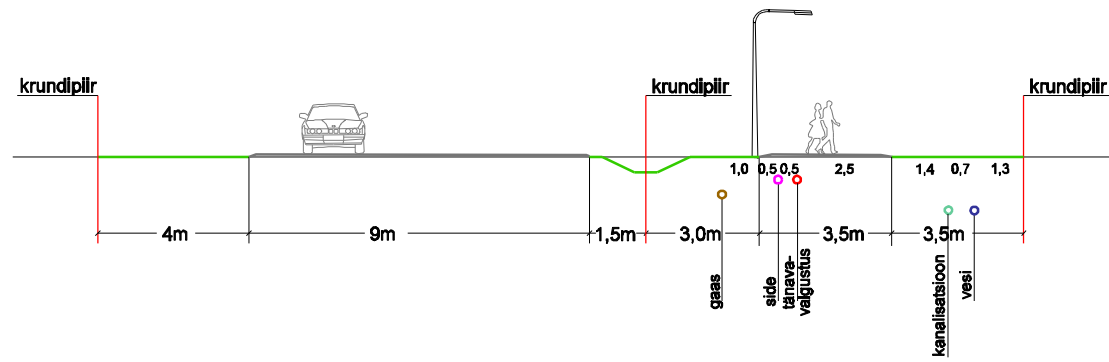
Lõige A - A
