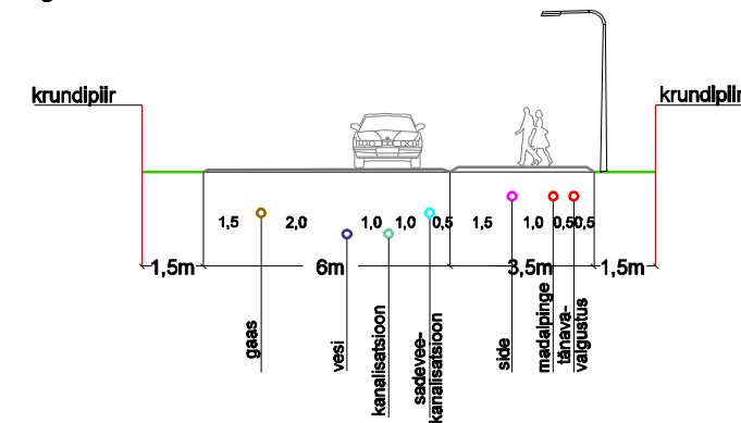
Lõige D - D
