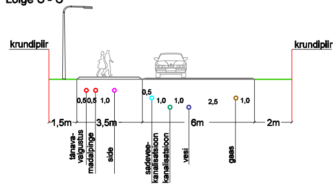
Lõige C - C
