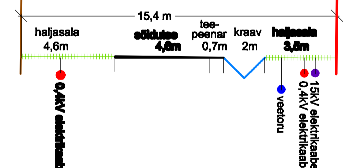
lõige C-C
