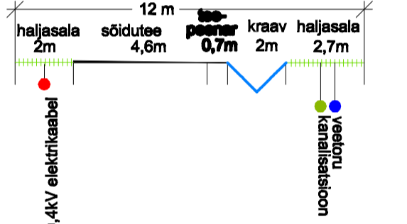
Teede ristprofiilid lõige A-A
