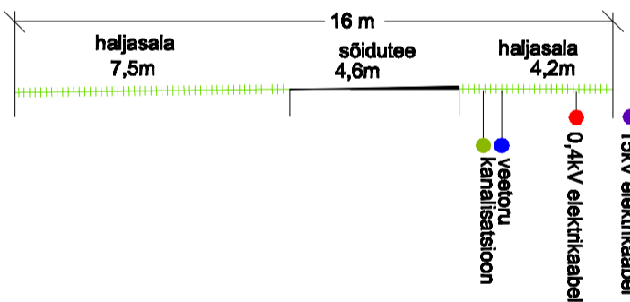
lõige B-B
