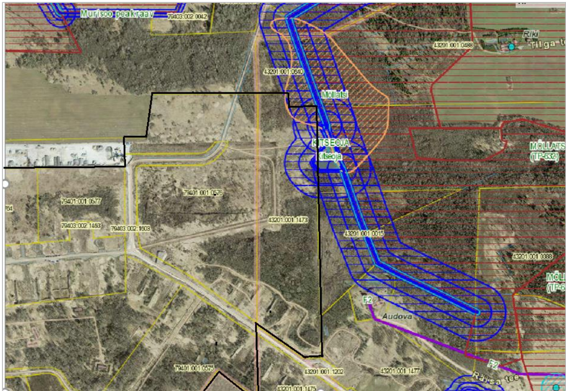
Joonis 7. Veekogudest tulenevad kalda kaitsevööndid vastavalt Maa-ameti kitsenduste rakendusele (musta joonega tähistatud planeeringuala ligikaudne piir).
