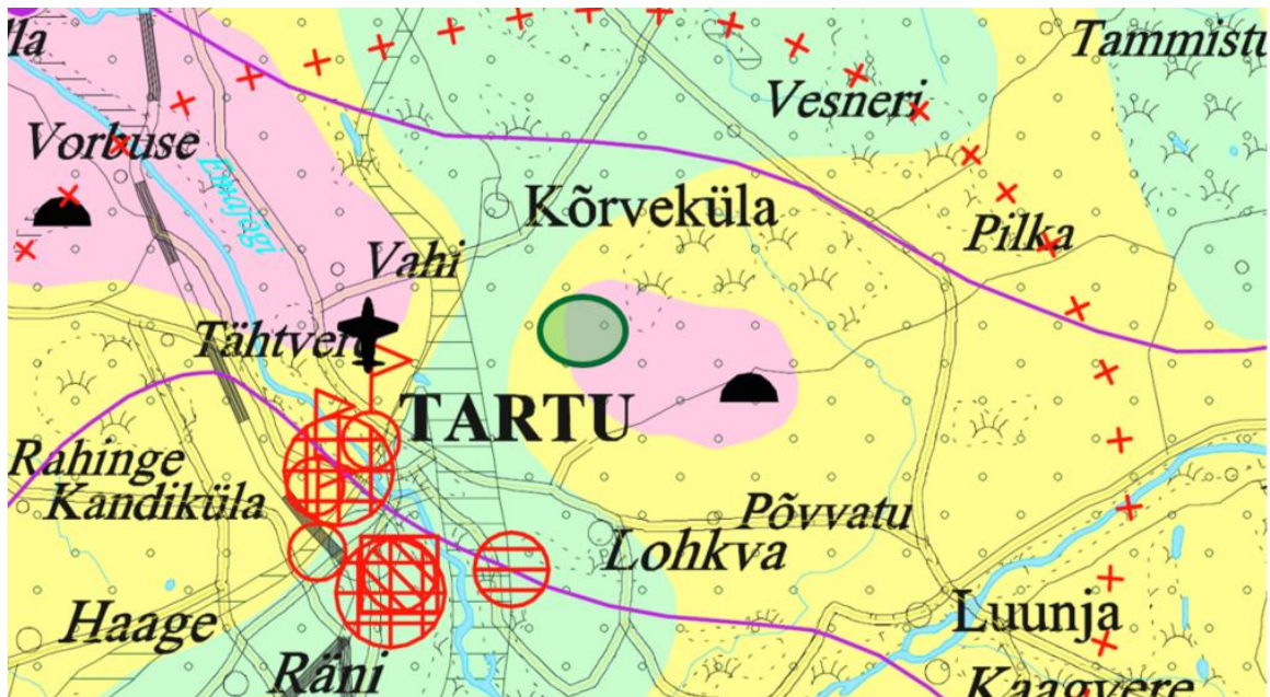
Joonis 11. Põhjavee kaitstus planeeringualal (planeeringuala ligikaudne asukoht on tähistatud rohelise ringiga).
