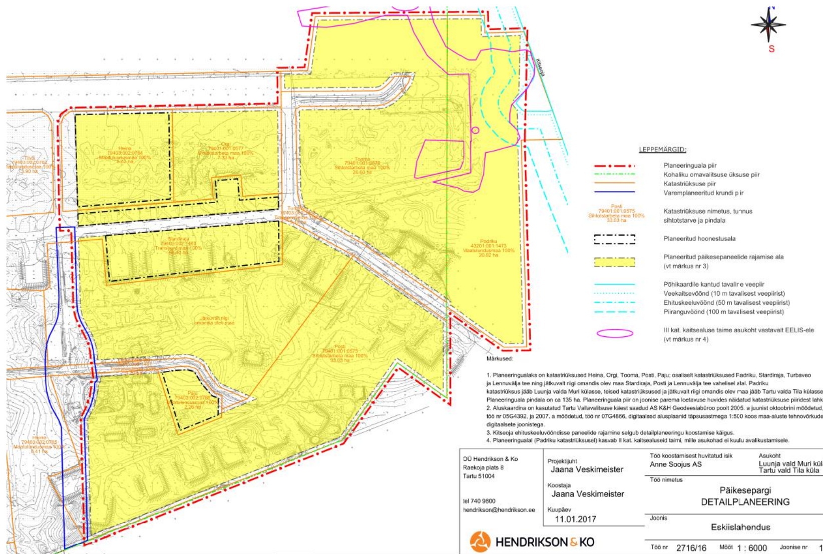
Skeem 1. Päikesepargi detailplaneeringu eskiis
